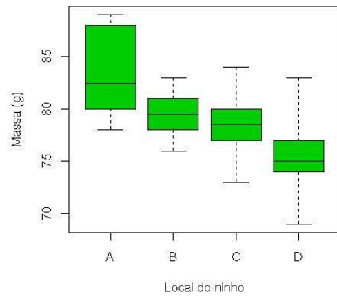
Figura 2. O mesmo boxplot sem os outliers da amostra D.
