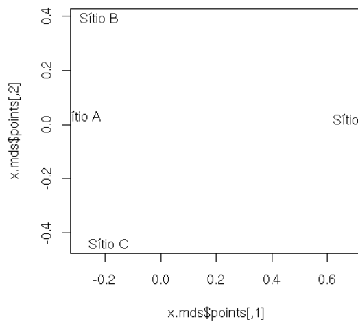
Figura 22. Ordinação nmMDS. Estresse<0.0001
