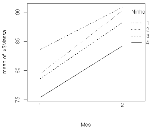
Figura 12. Gráfico de interação: a variação na massa média entre os locais é parecida entre os dois meses.
