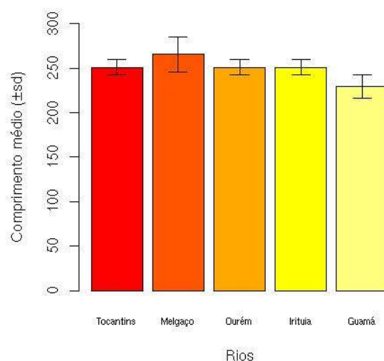
Figura 6. Média ( \pm desvio padrão) dos dados (larvas.csv) sobre comprimento de larvas de bivalves de água doce em cinco diferentes rios amazônicos.
